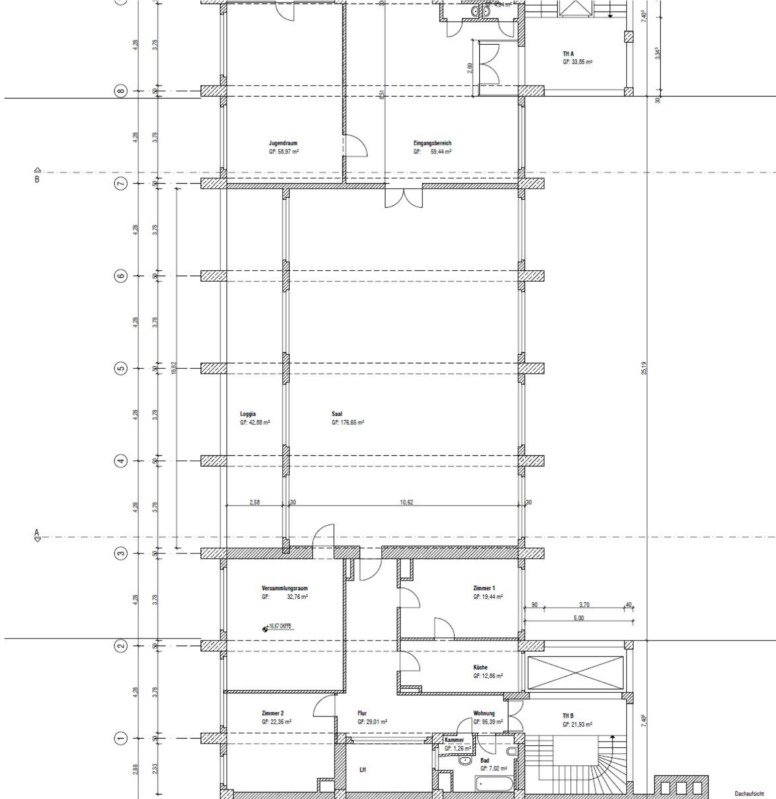
Dachaufsicht
