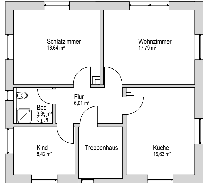
Grundriss Obergeschoss
