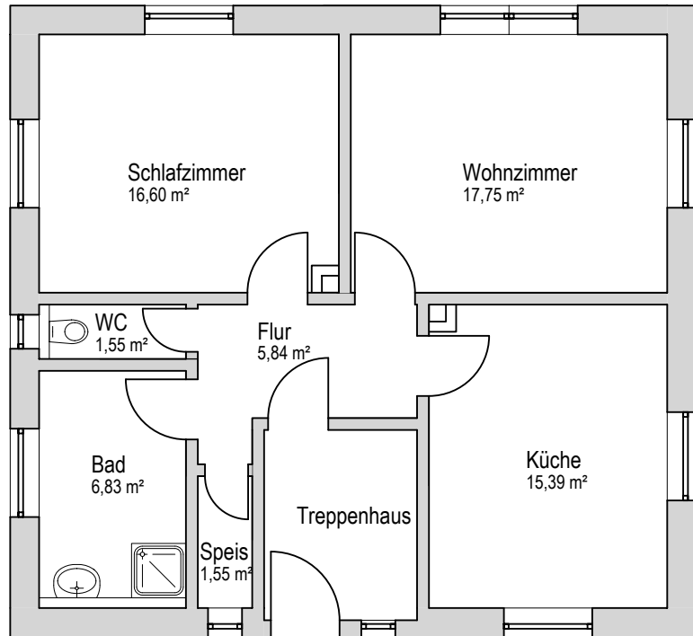
Grundriss Erdgeschoss
