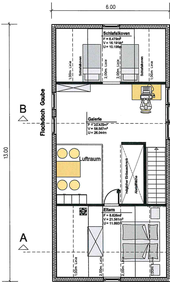
Dachgeschoss
