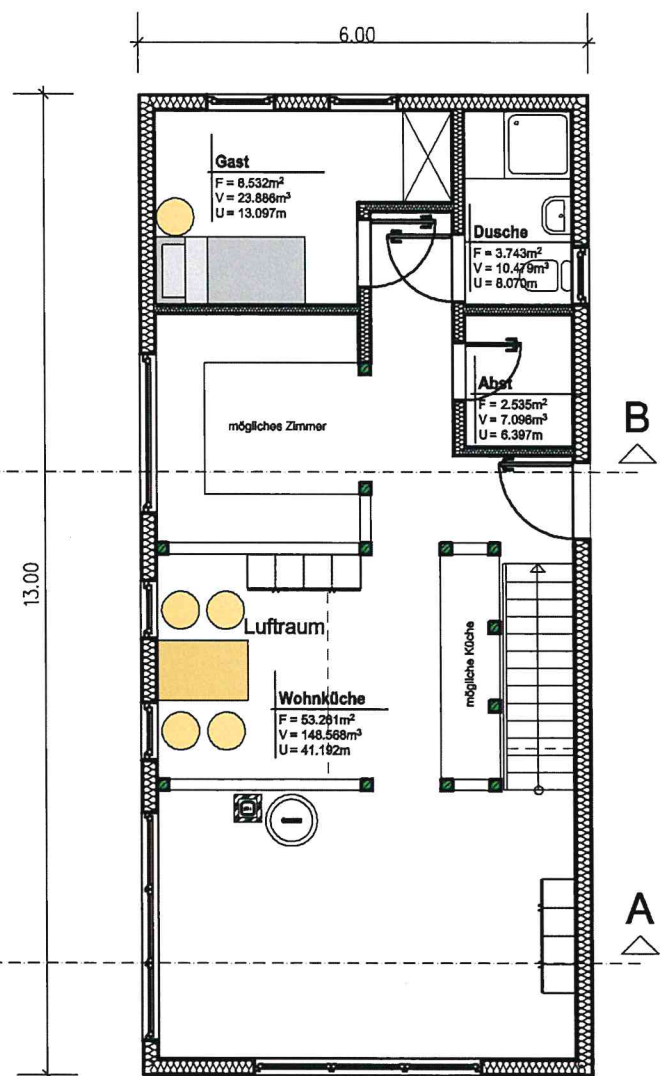
Erdgeschoss
