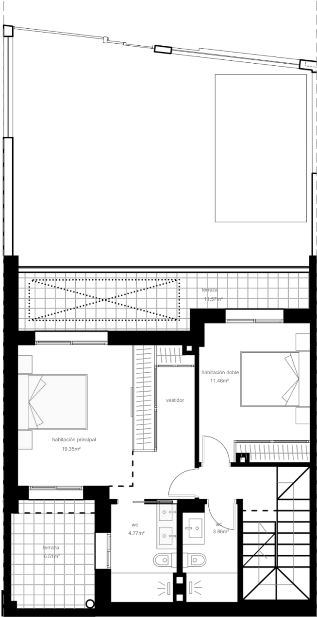
PLANTA PRIMERA
