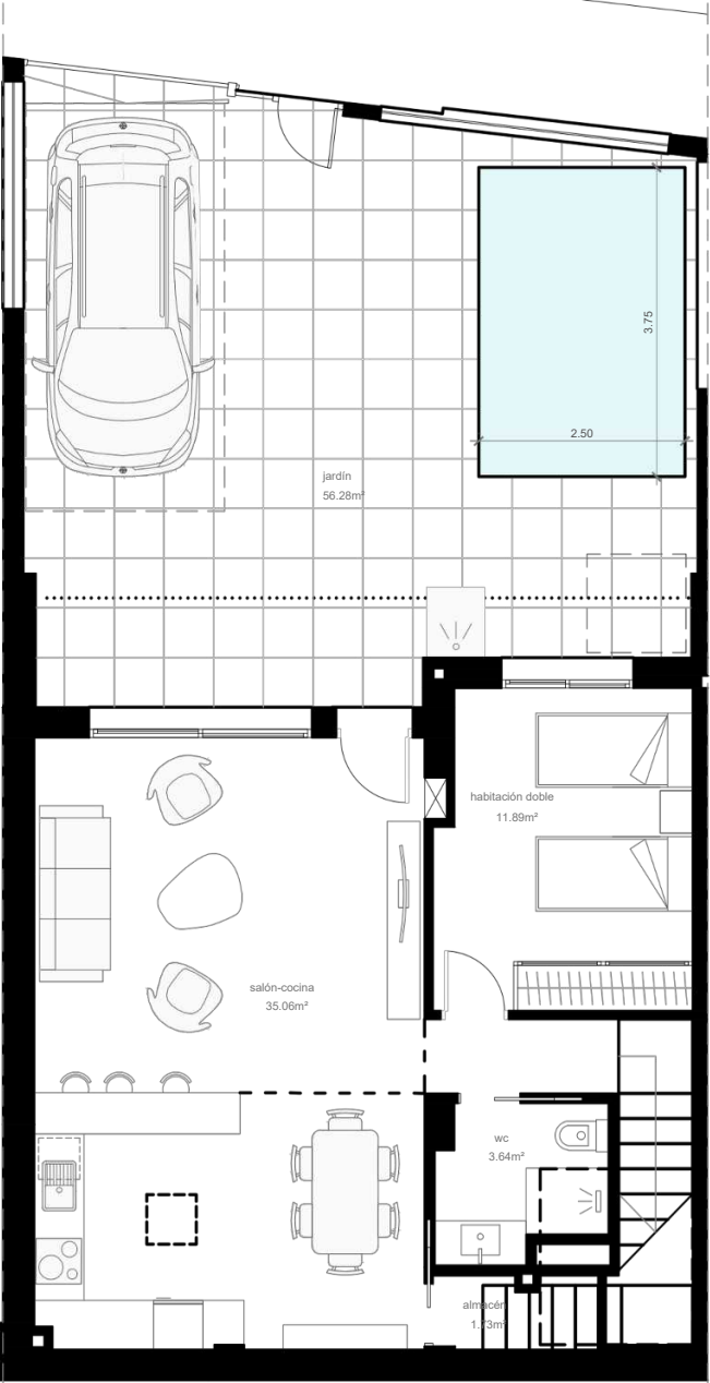
PLANTA BAJA
