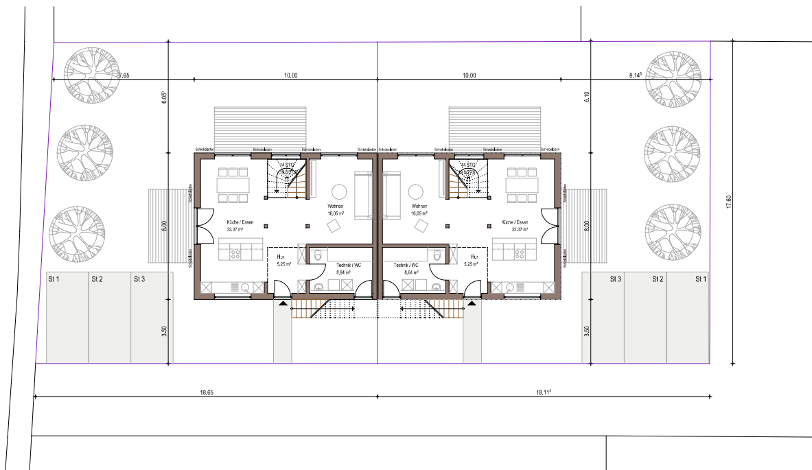
ERDGESCHOSS
