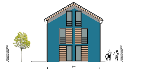
ANSICHT NORD-SÜD
