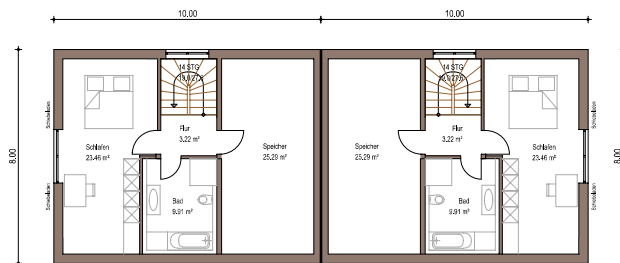
DACHGESCHOSS
