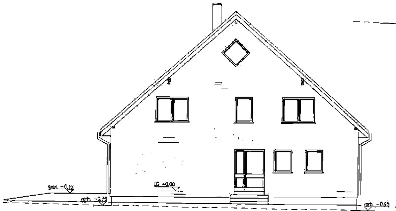
Ansicht Norden
