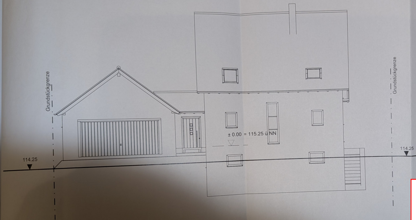
Nord - Ansicht
