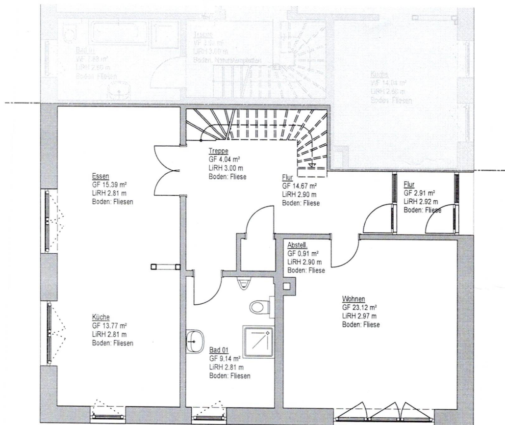
Grundriss Erdgeschoss M 1:100
