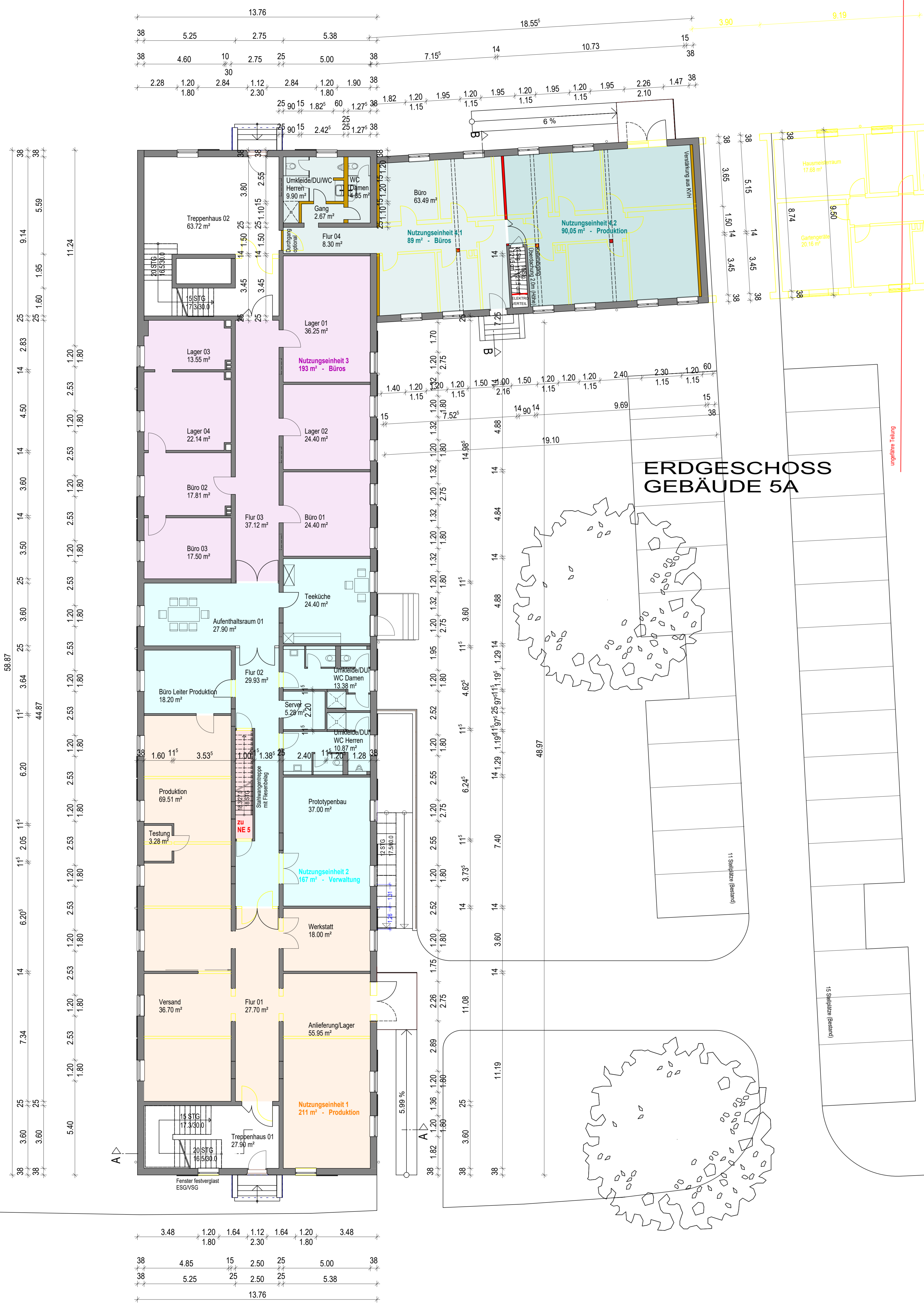
ERDGESCHOSS GEBÄUDE 5
