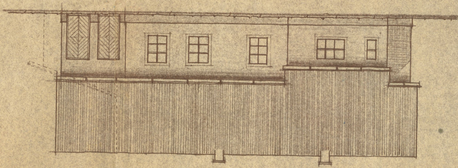
ANSICHT - WEST
