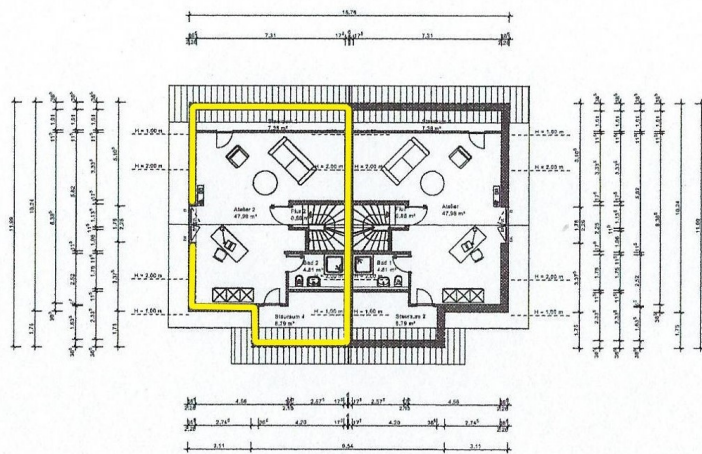
DACHGESCHOSS Grundriss
