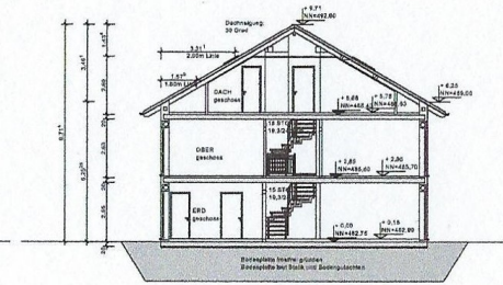
SNITT A - 1
