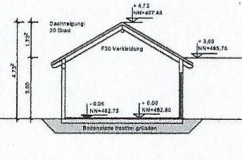
SNITT C - 1
