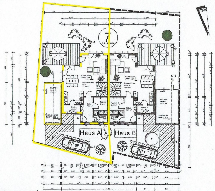
ERDGESCHOSS Grundriss
