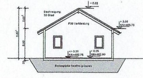
SNITT B - 1
