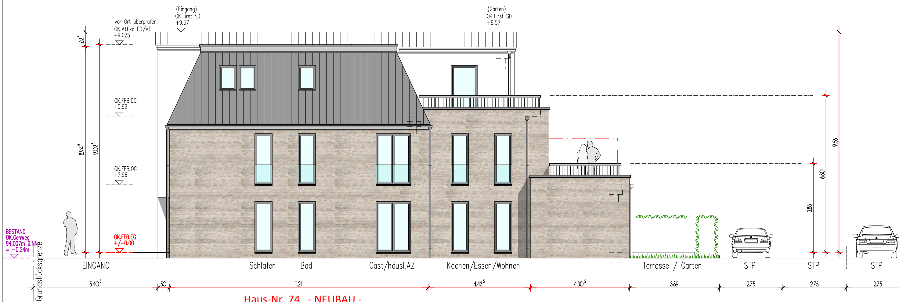
Ansicht: Nord-West | Seitenansicht
