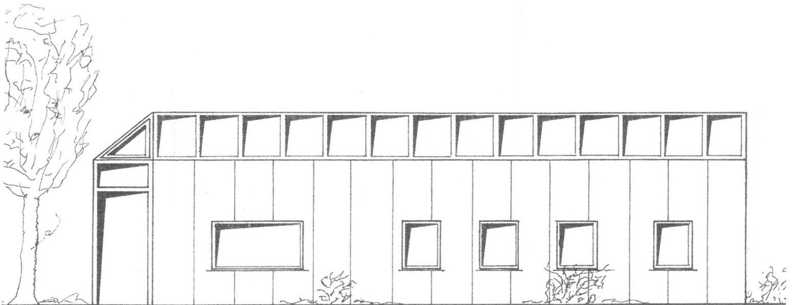
ANSICHT VON OSTEN
