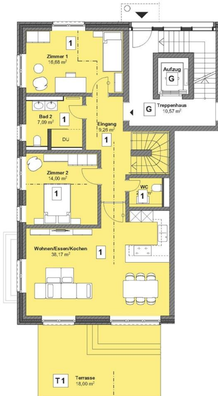
Erdgeschoss - Wohnung 1
