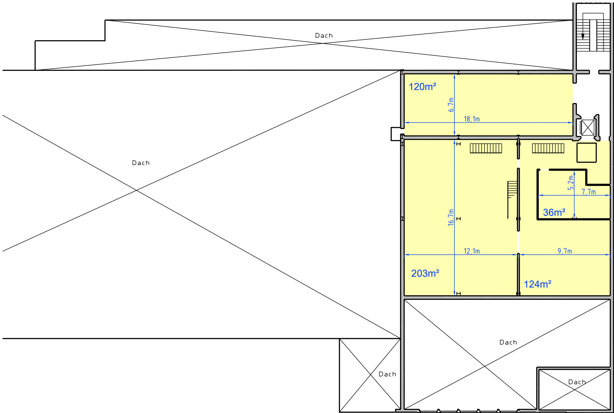
4. Obergeschoss
