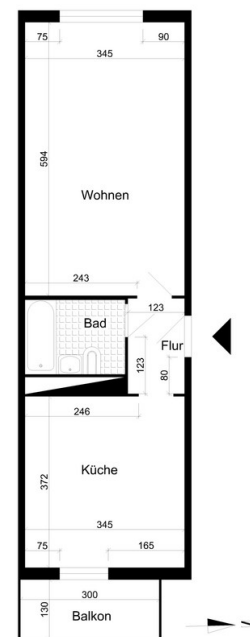
Grundriss
