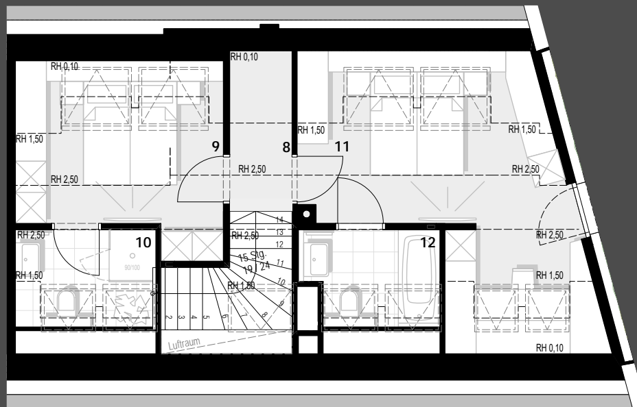
2. DACHGESCHOSS
