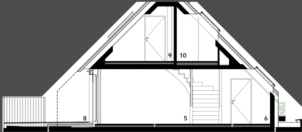
QUERSCHNITT
