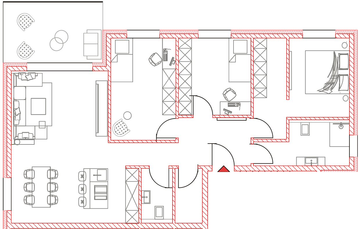
Grundriss zeigt Wohnung C 0.2
