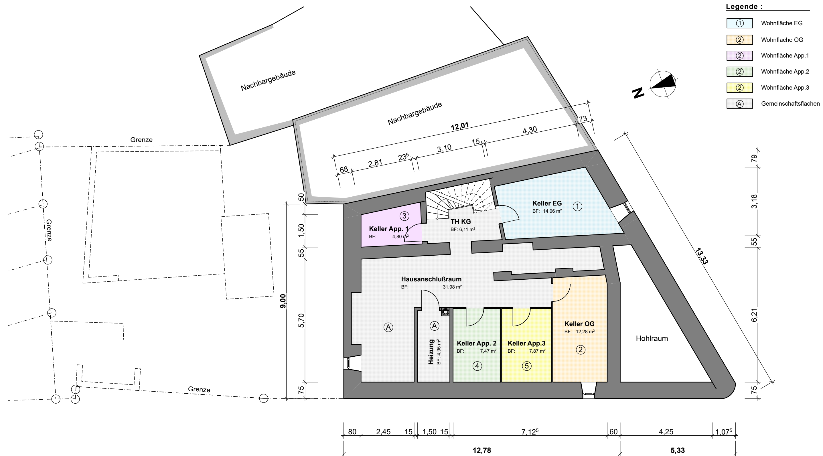
KELLERGECHOSS M = 1 : 100
