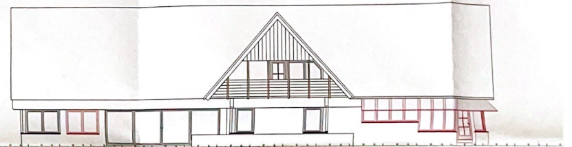
ANSICHT SÜD-OST M. 1:100
