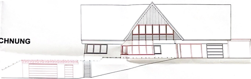
ANSICHT NORD-OST M. 1:100
