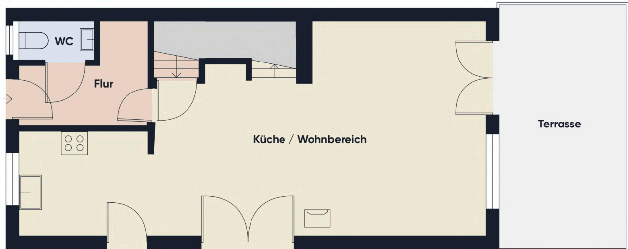
Grundrissplan ohne Maßstab EG
