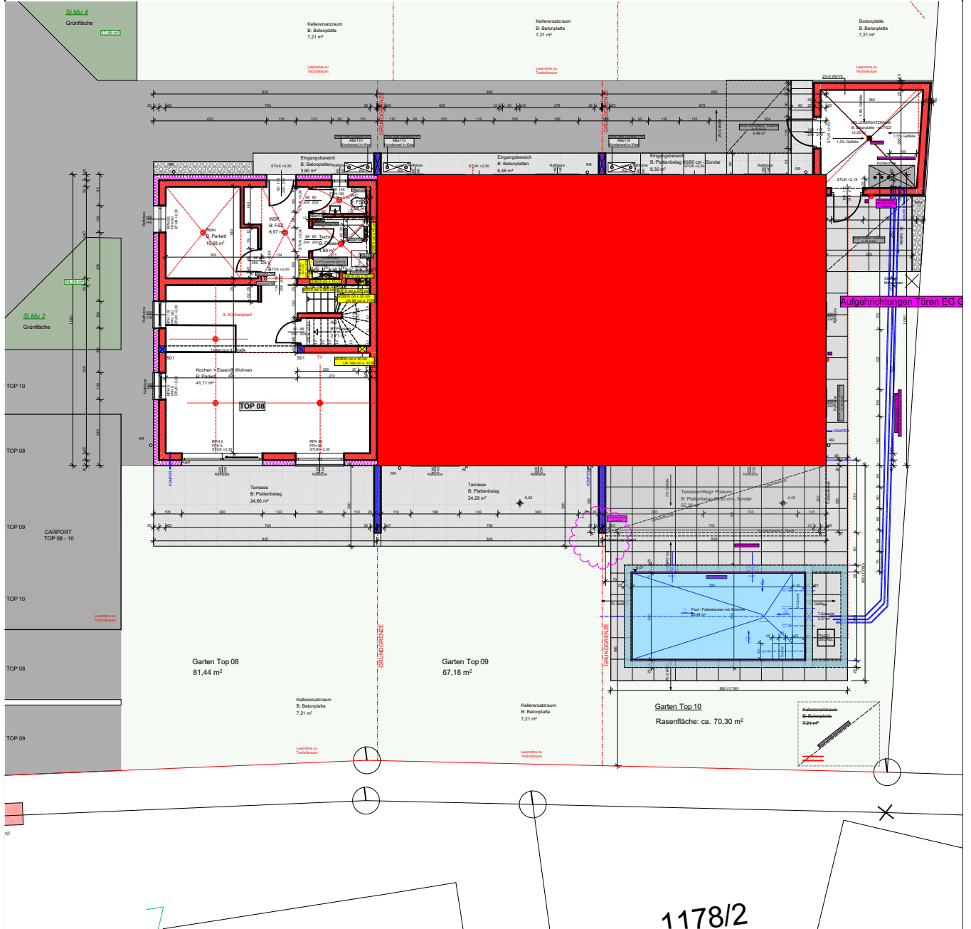
Übersichtsplan - M 1:200
