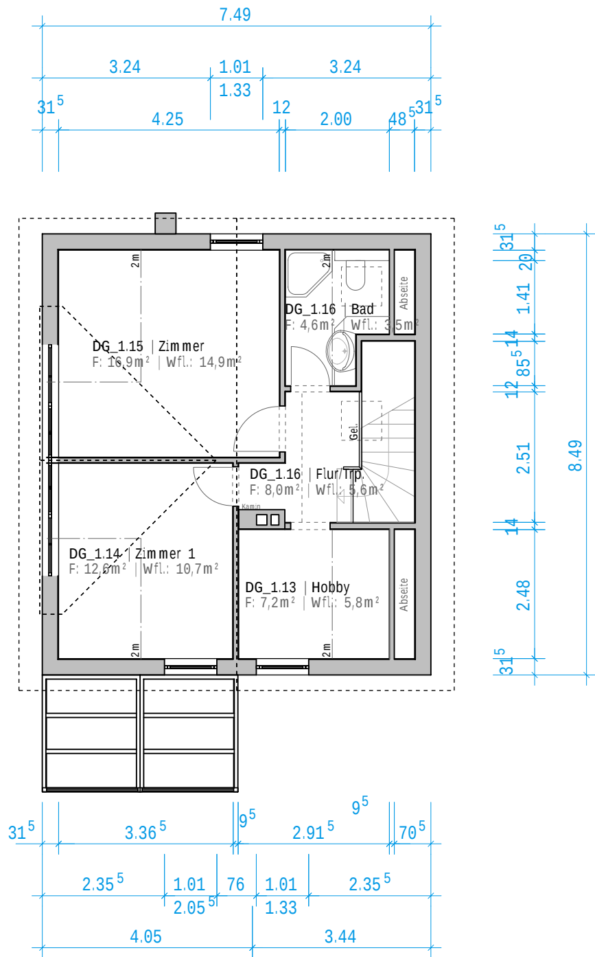
Grundriss Dachgeschoss
