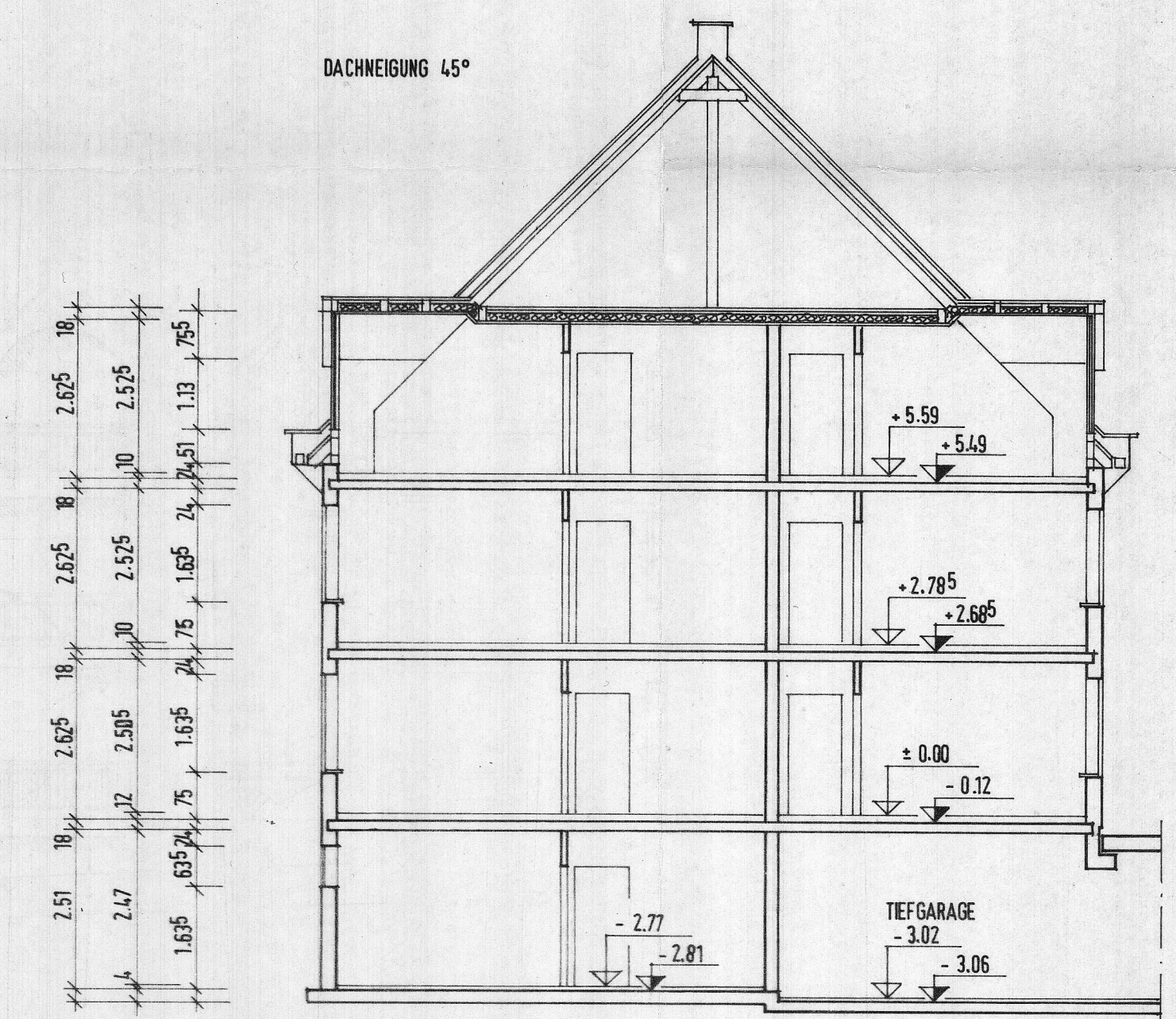
SCHNITT D-D
