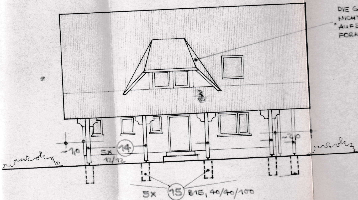
NORDANSICHT (neu)
