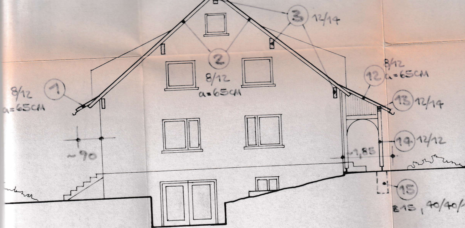
OSTANSICHT (neu)
