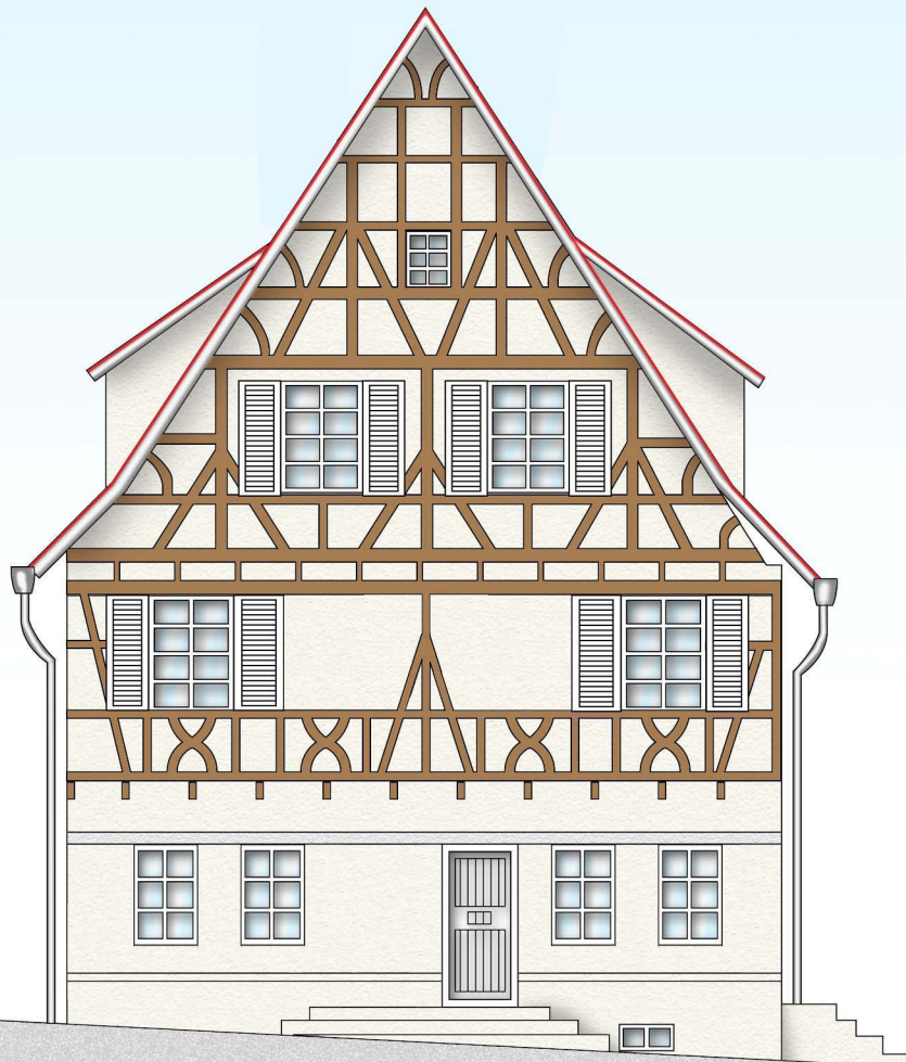
Ansicht - Strasse
