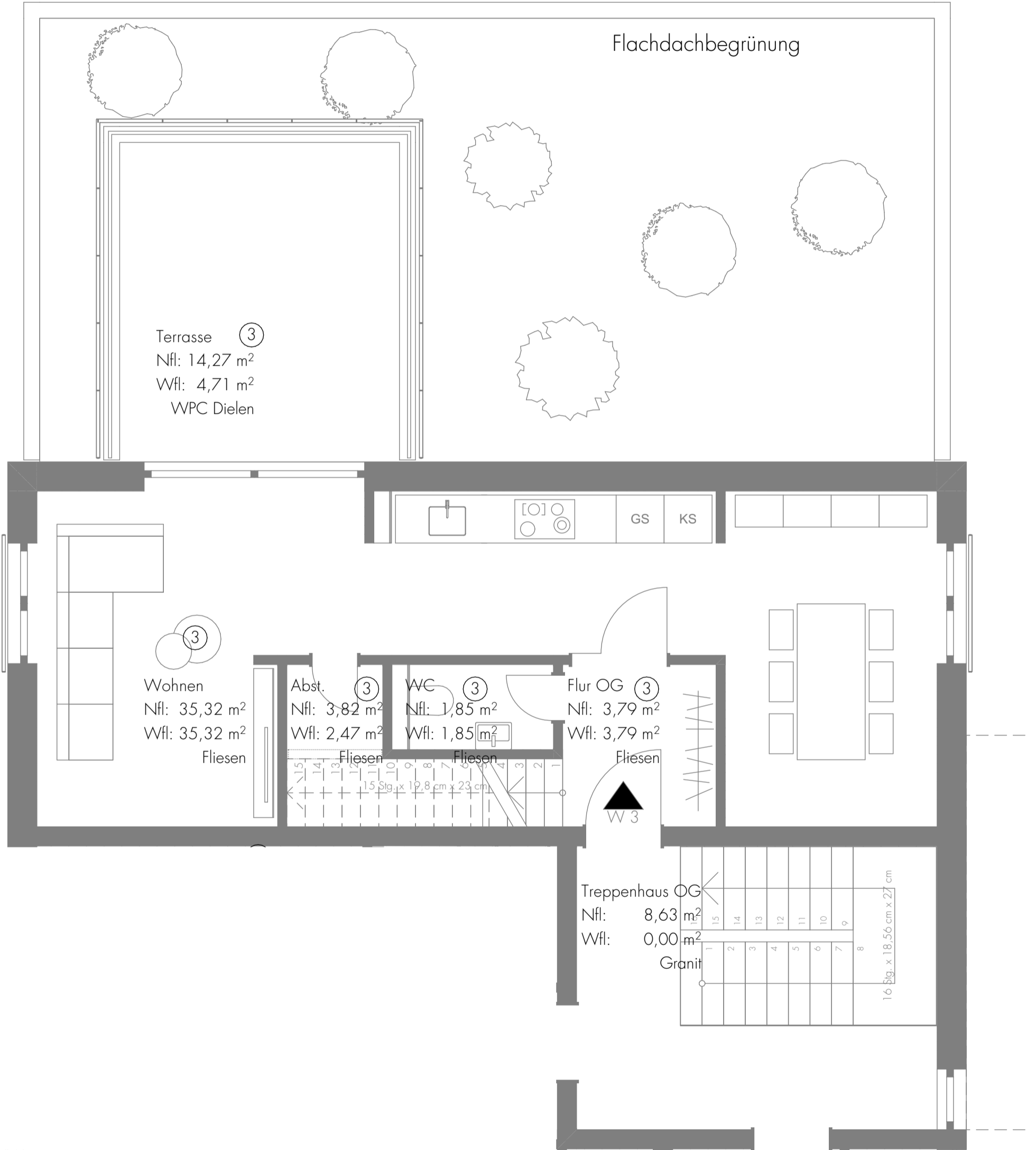
Wohnung 3 Obergeschoss
