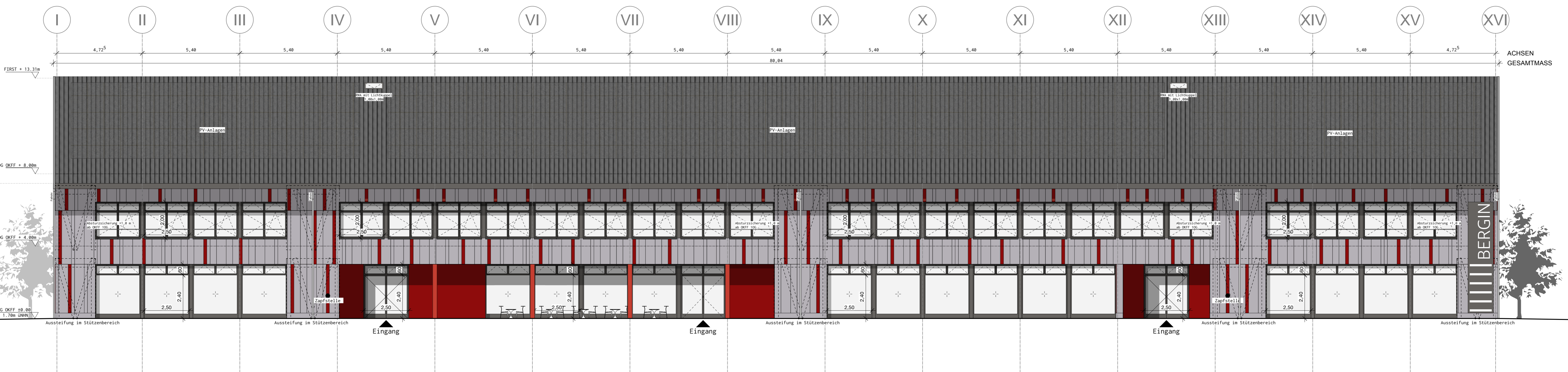
Ansicht Süd
