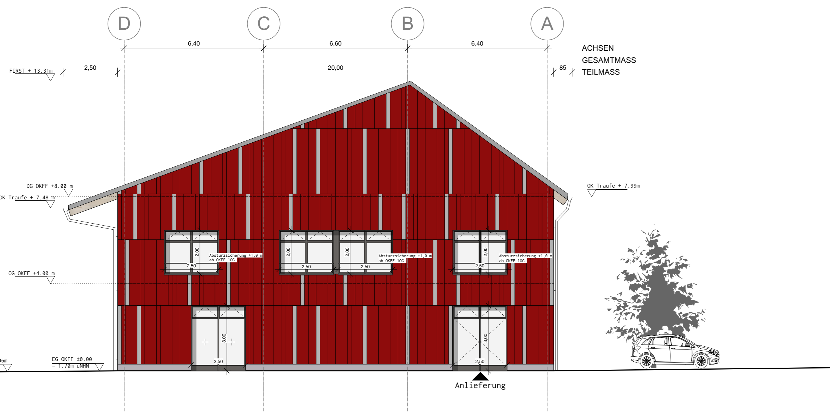
Ansicht Ost schematisch Geschäftshaus 1
