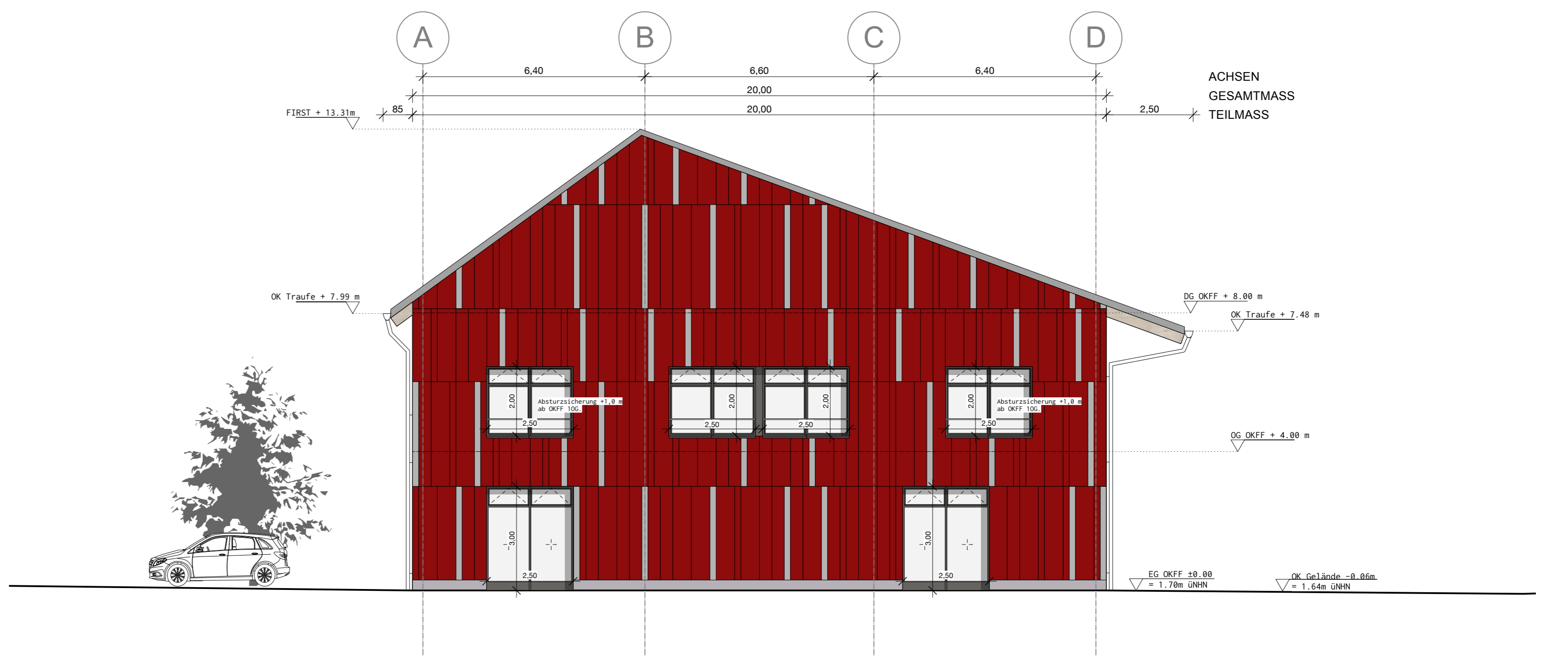
Ansicht West schematisch Geschäftshaus 1
