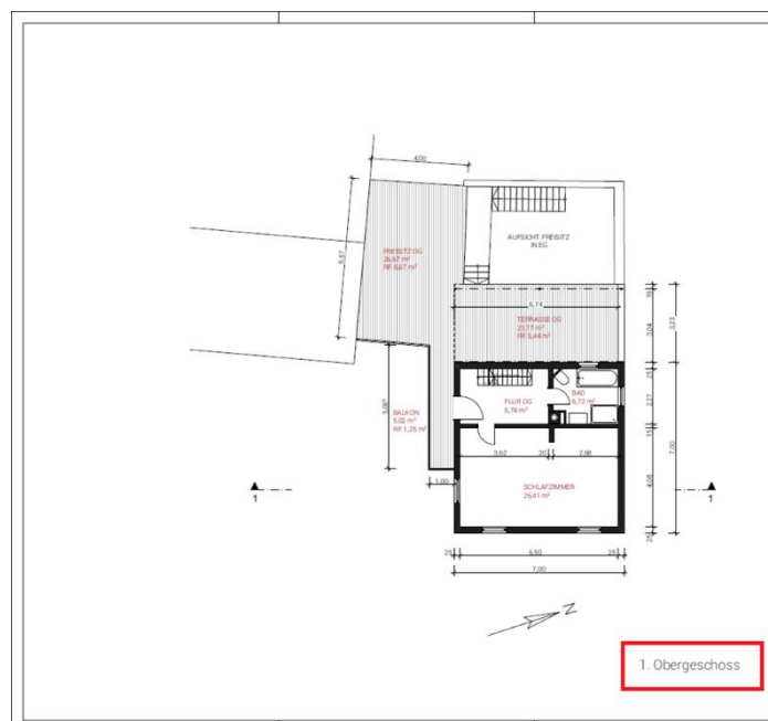
Grundrisse OG
