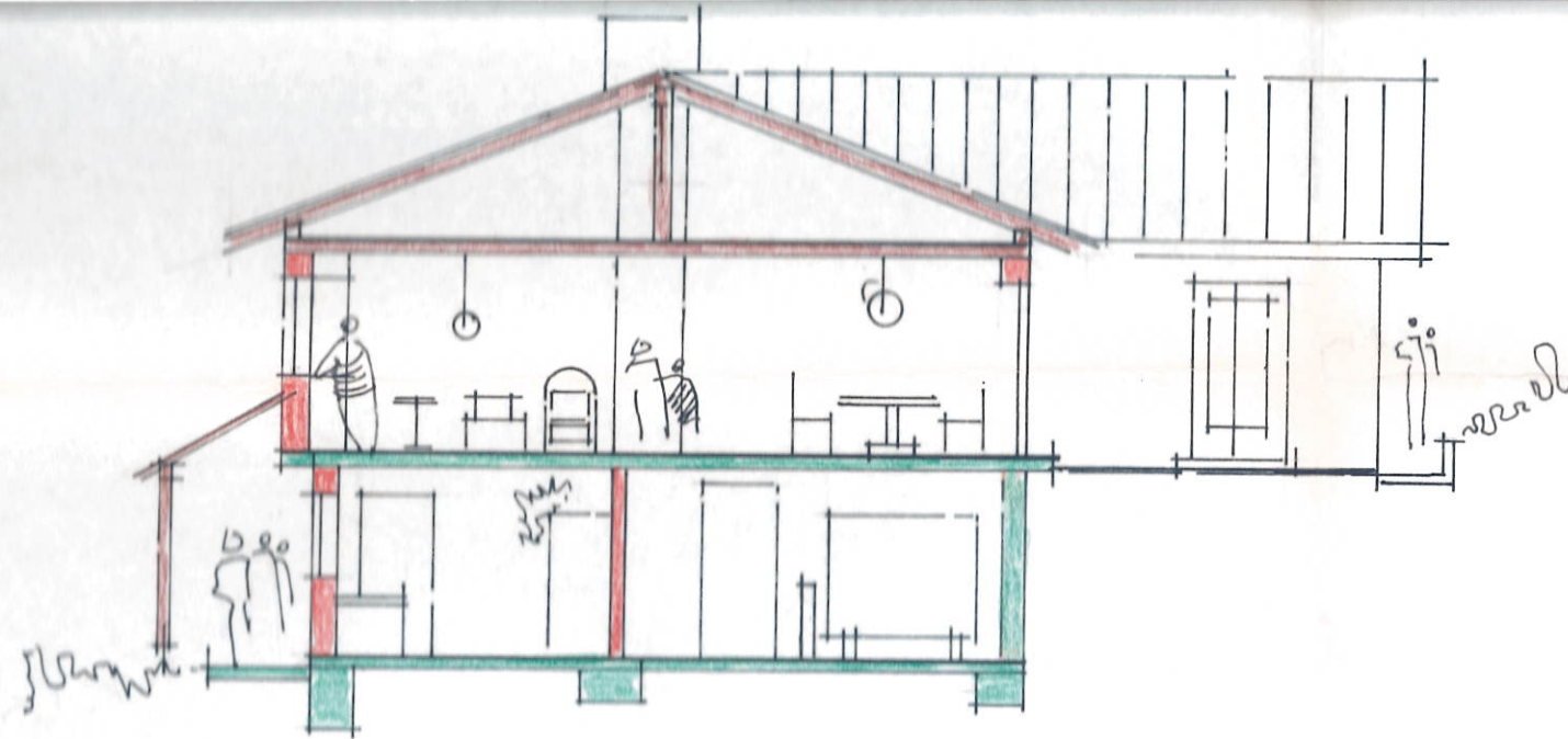
schnitt a
