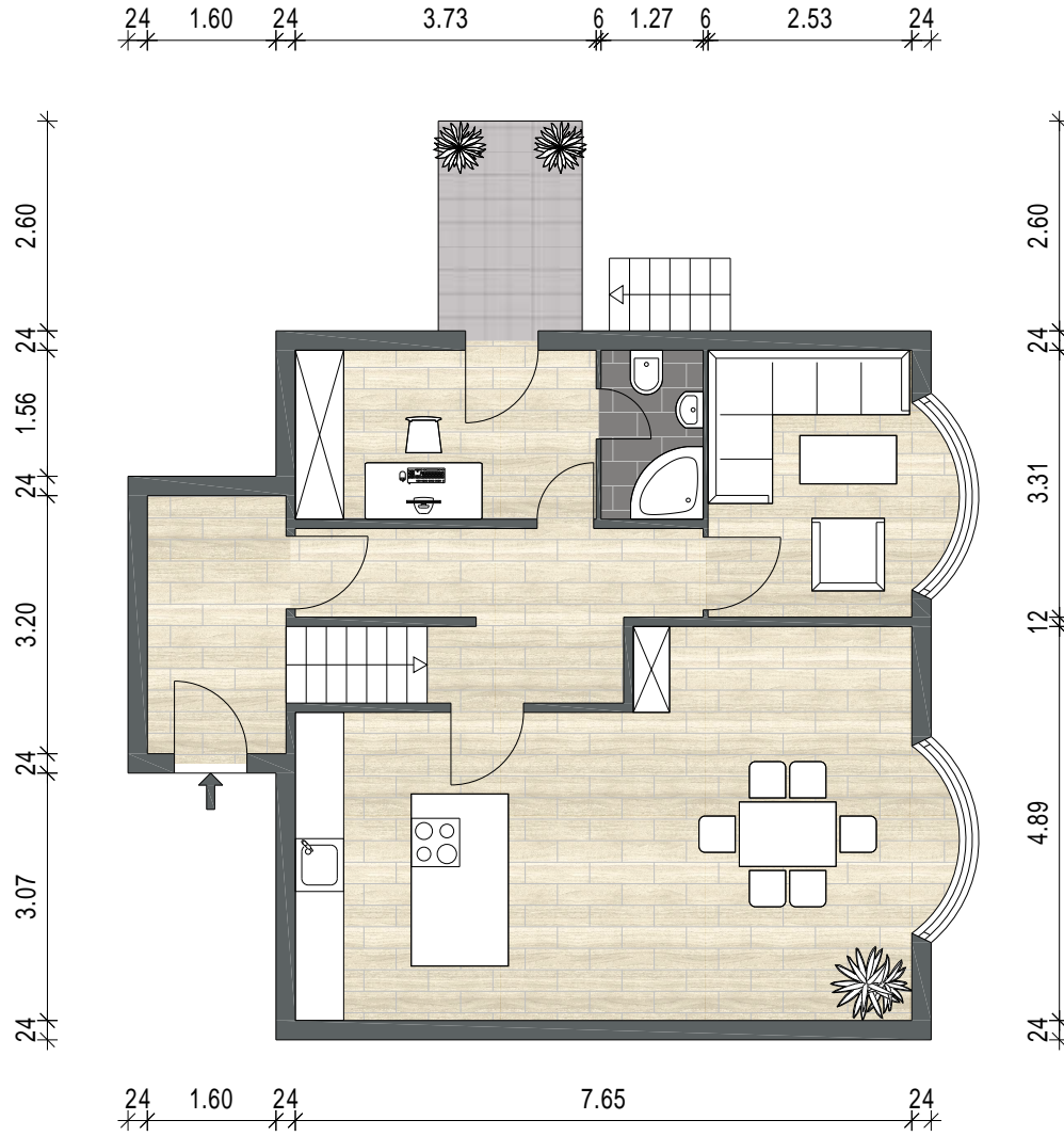
Erdgeschoss
