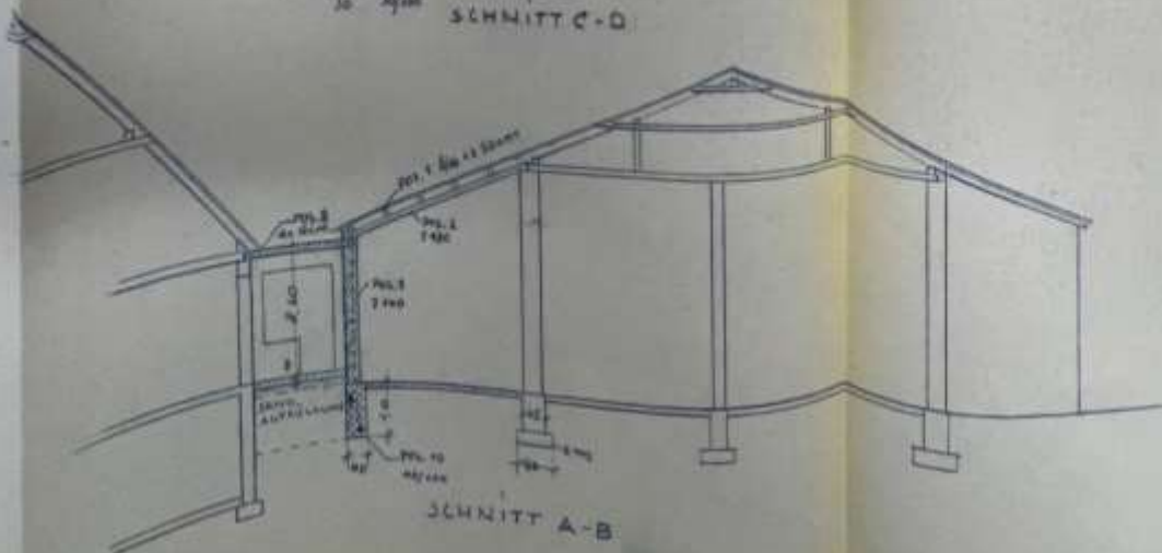
SCHNITT C-D
