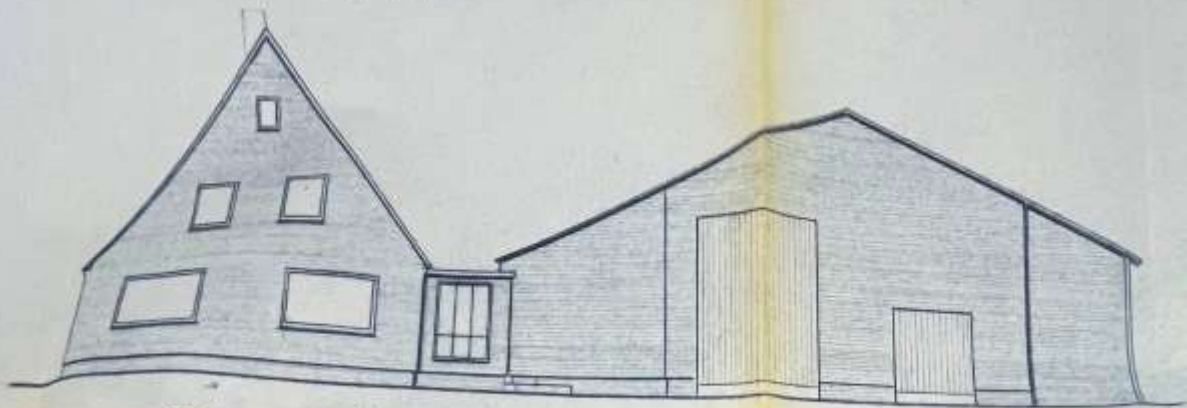
STRASSEN-ANSICHT-SÜDEN
