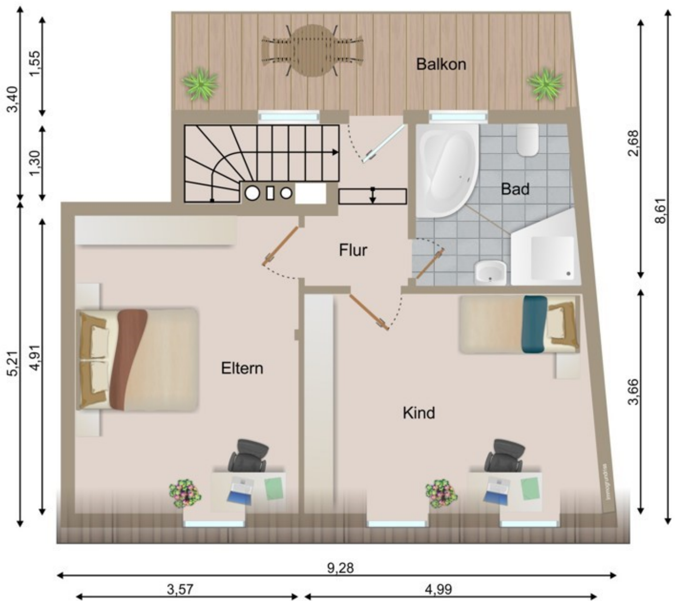
Obergeschoss
