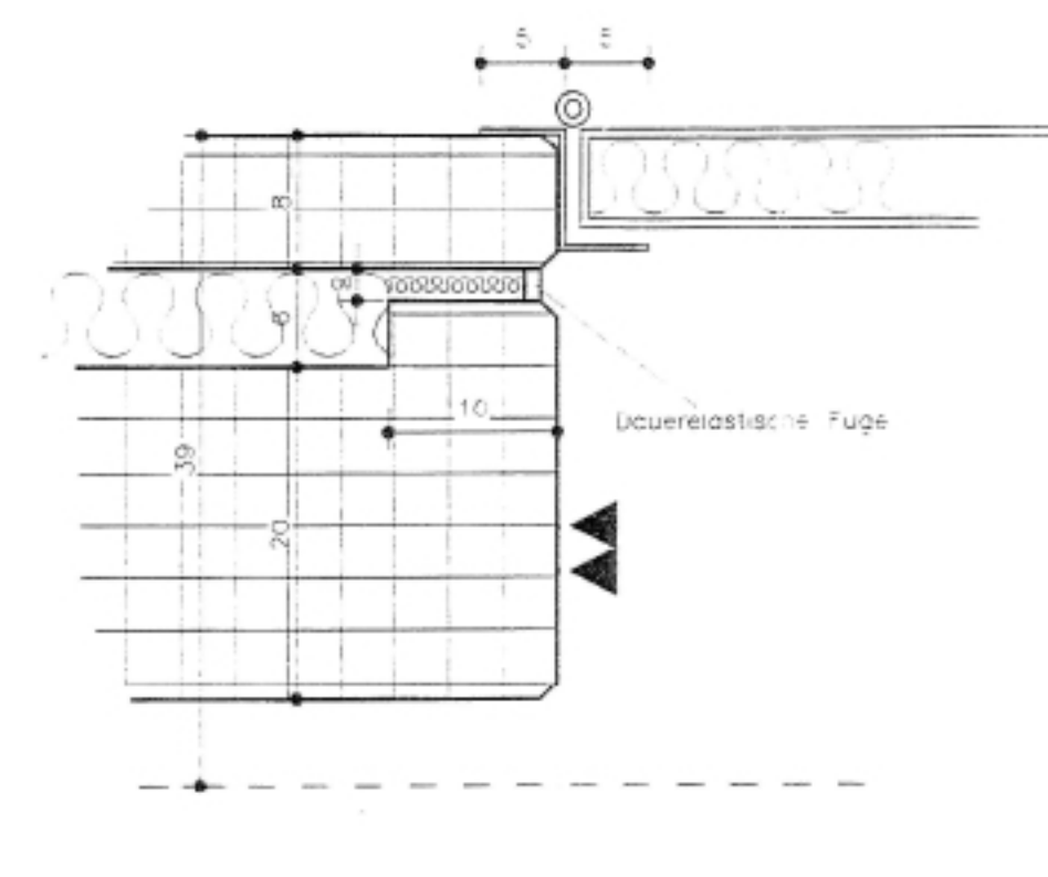
Detail : Tür 1:5
