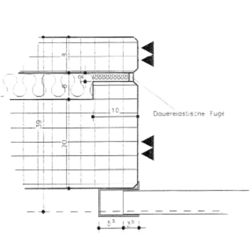
Detail : Sektionaltor 1:5
