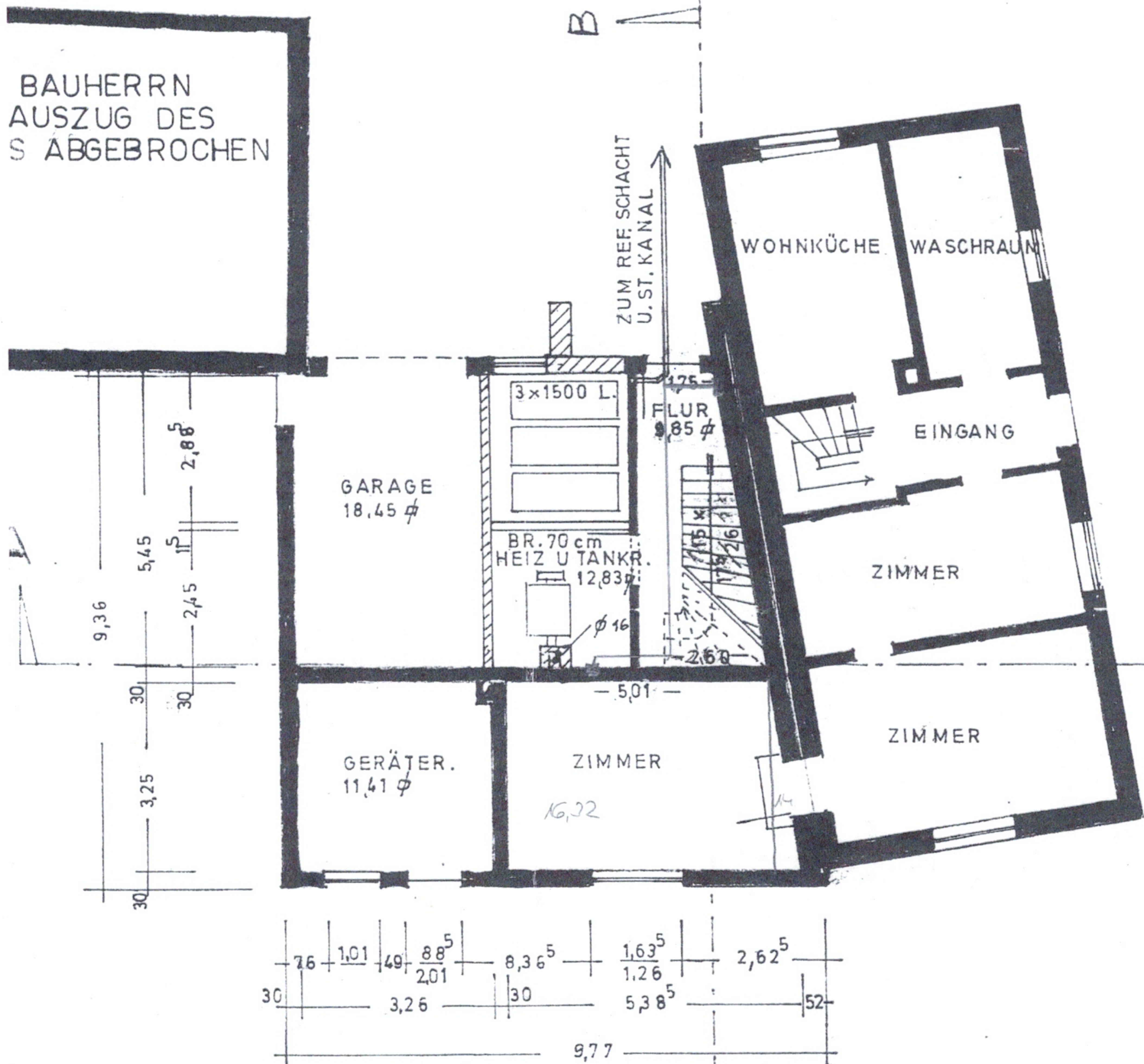
GRUNDRISS ERDGESCHOSS
