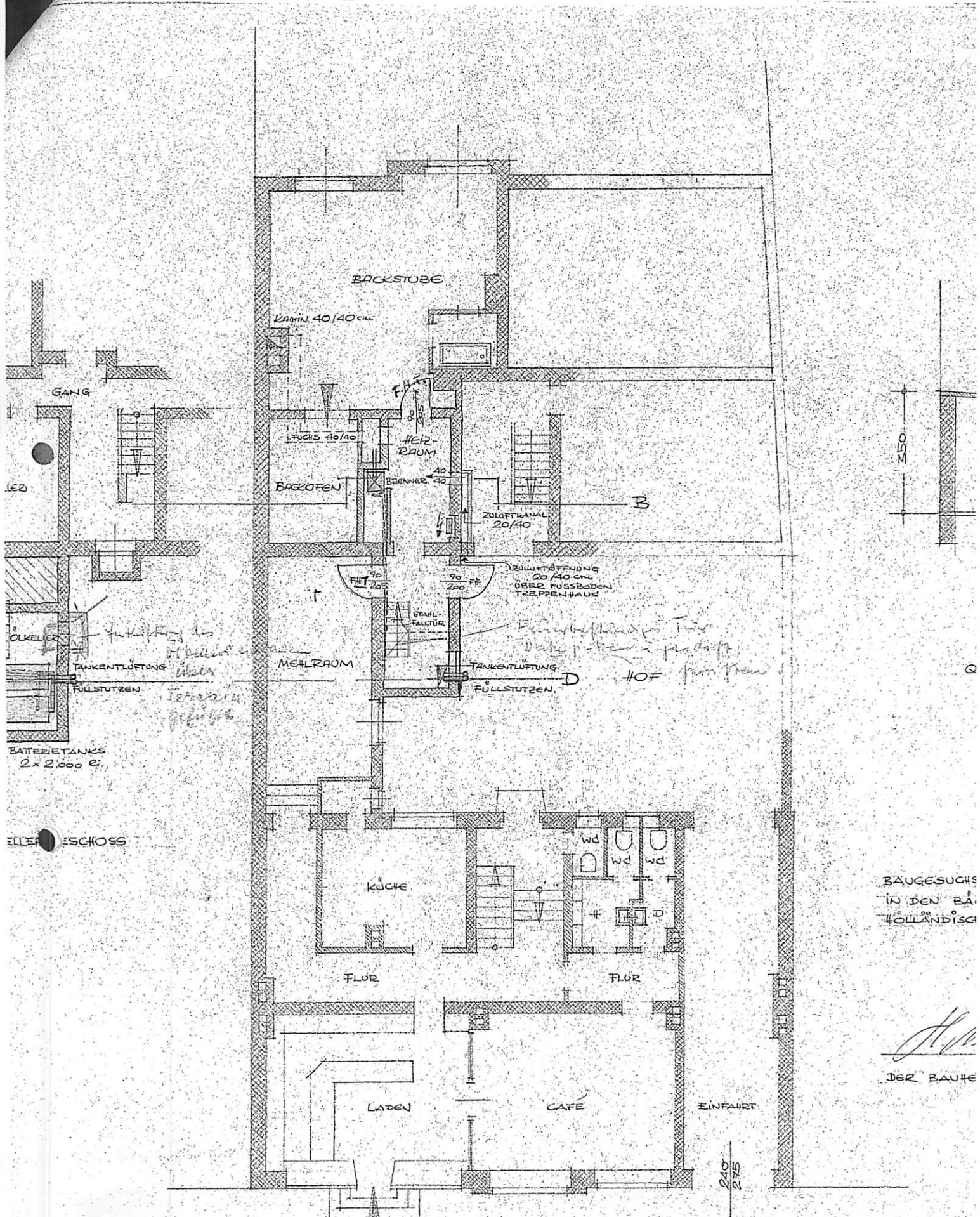
GRUNDRISS ERDGESCHOSS M = 1 = 100 NACH BAUGESUCHSZEICHNUNG BP 2179/47 ERGÄNZT DURCH ÖRTL. AUFMASS.
