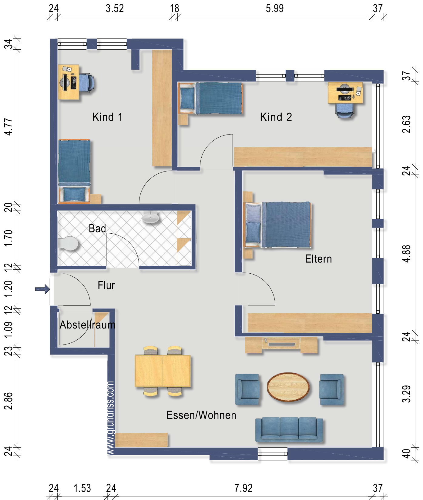
Erdgeschoss
