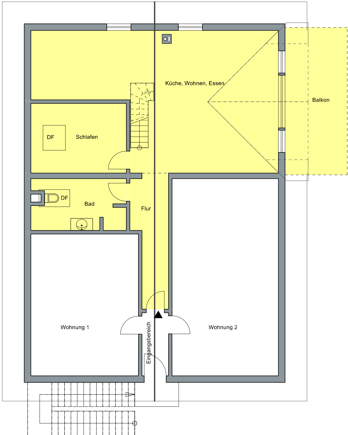
Grundriss Obergeschoss
