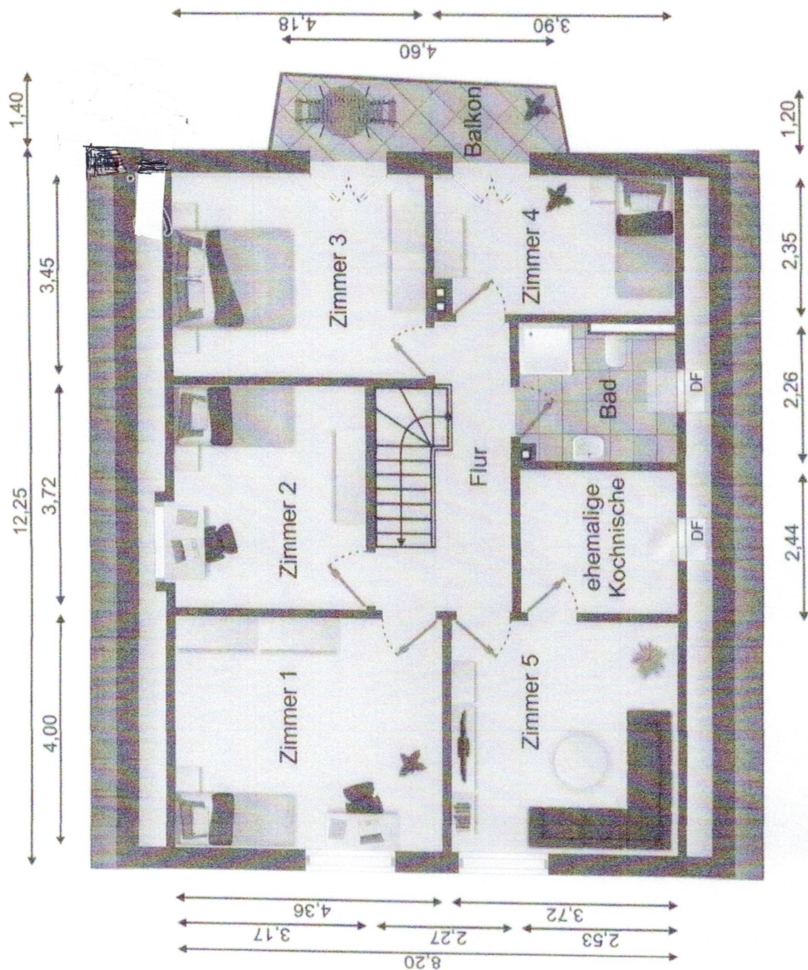
Dachgeschoss
