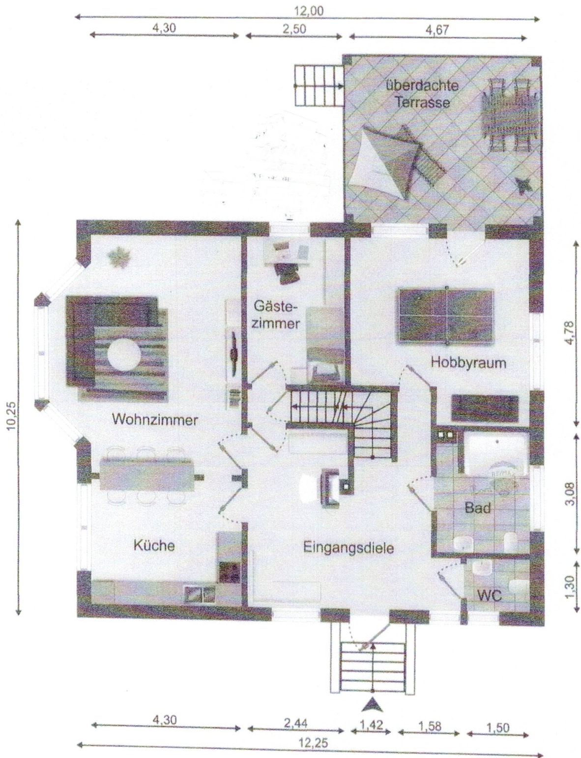
Erdgeschoss
