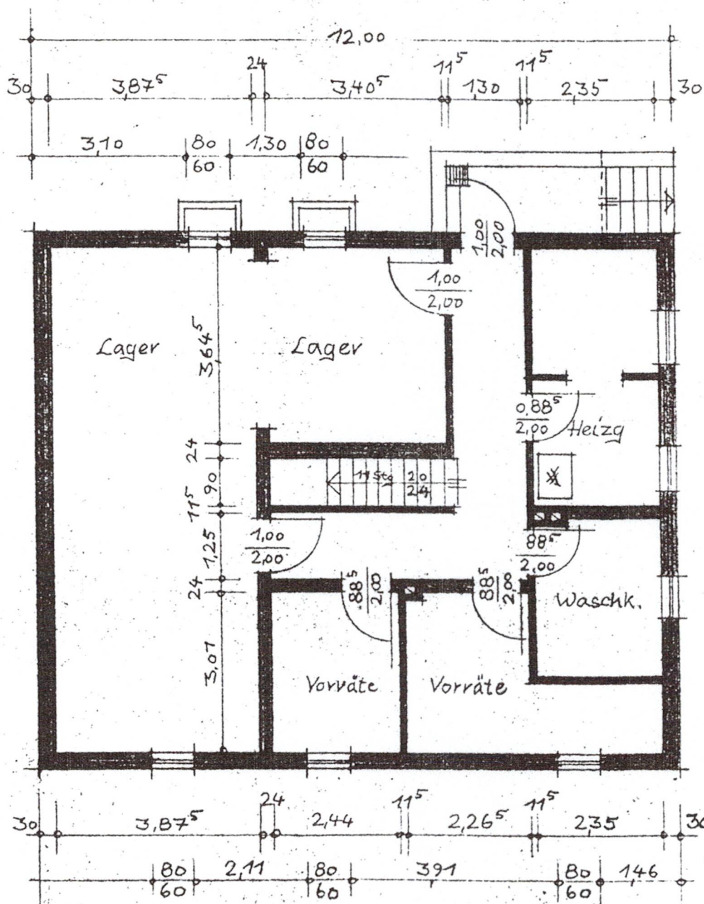
Kellergeschoss
