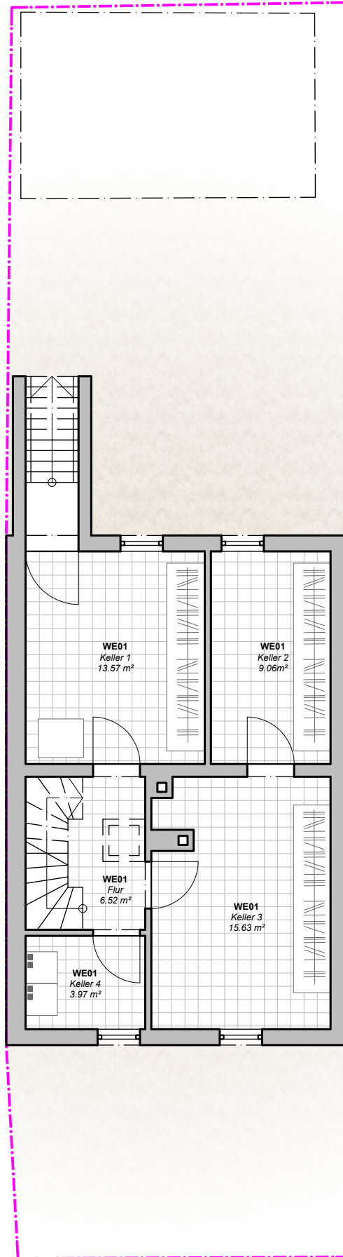
Grundriss Kellergeschoss
