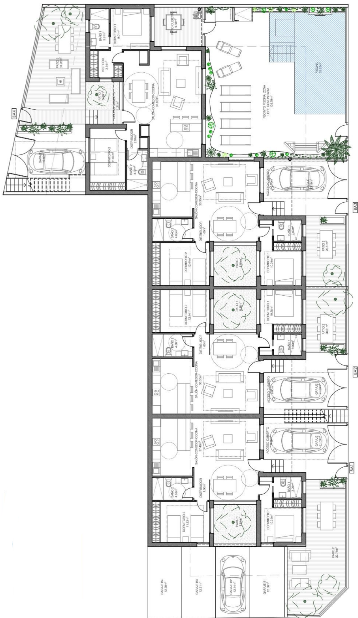
PLANTA BAJA
