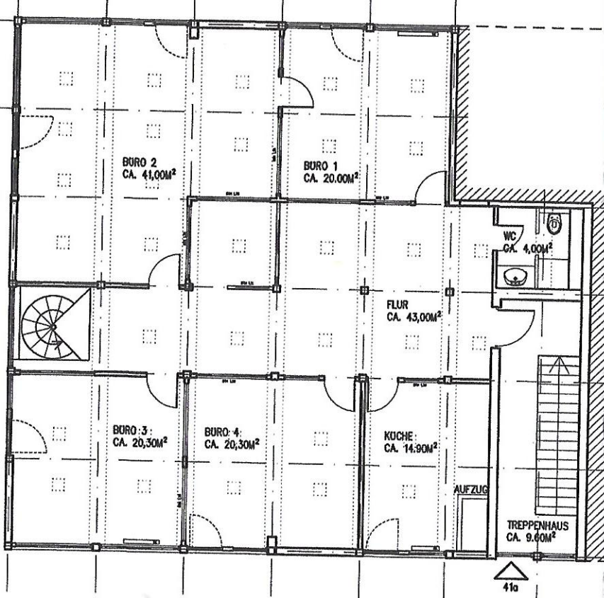
GRUNDRISS 1. OG M.1: 100
