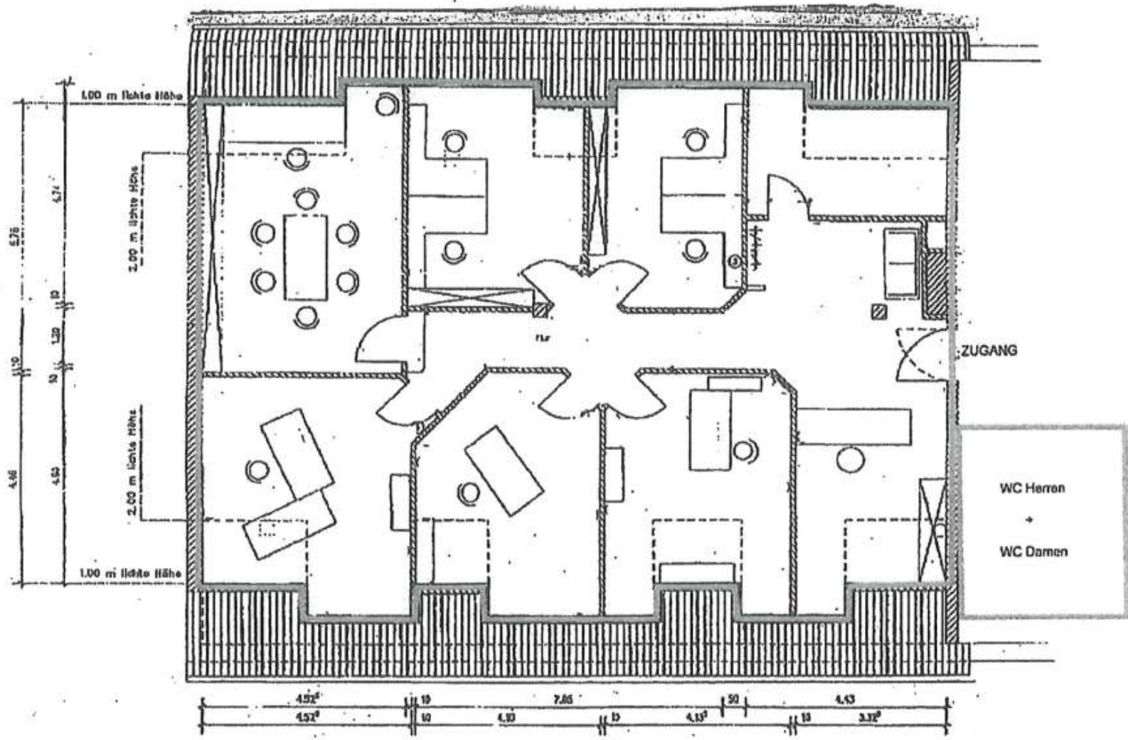
DACHGESCHOSS M: 1:100
