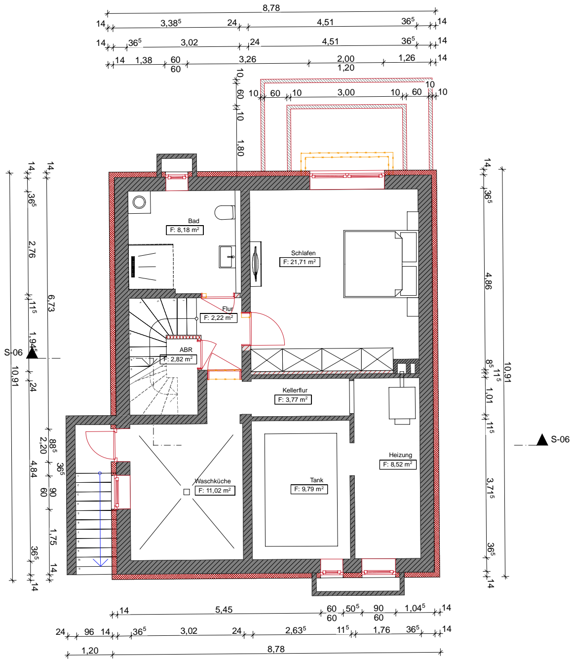
Kellergeschoss Nachbar Am Strasserfeld 1:100
