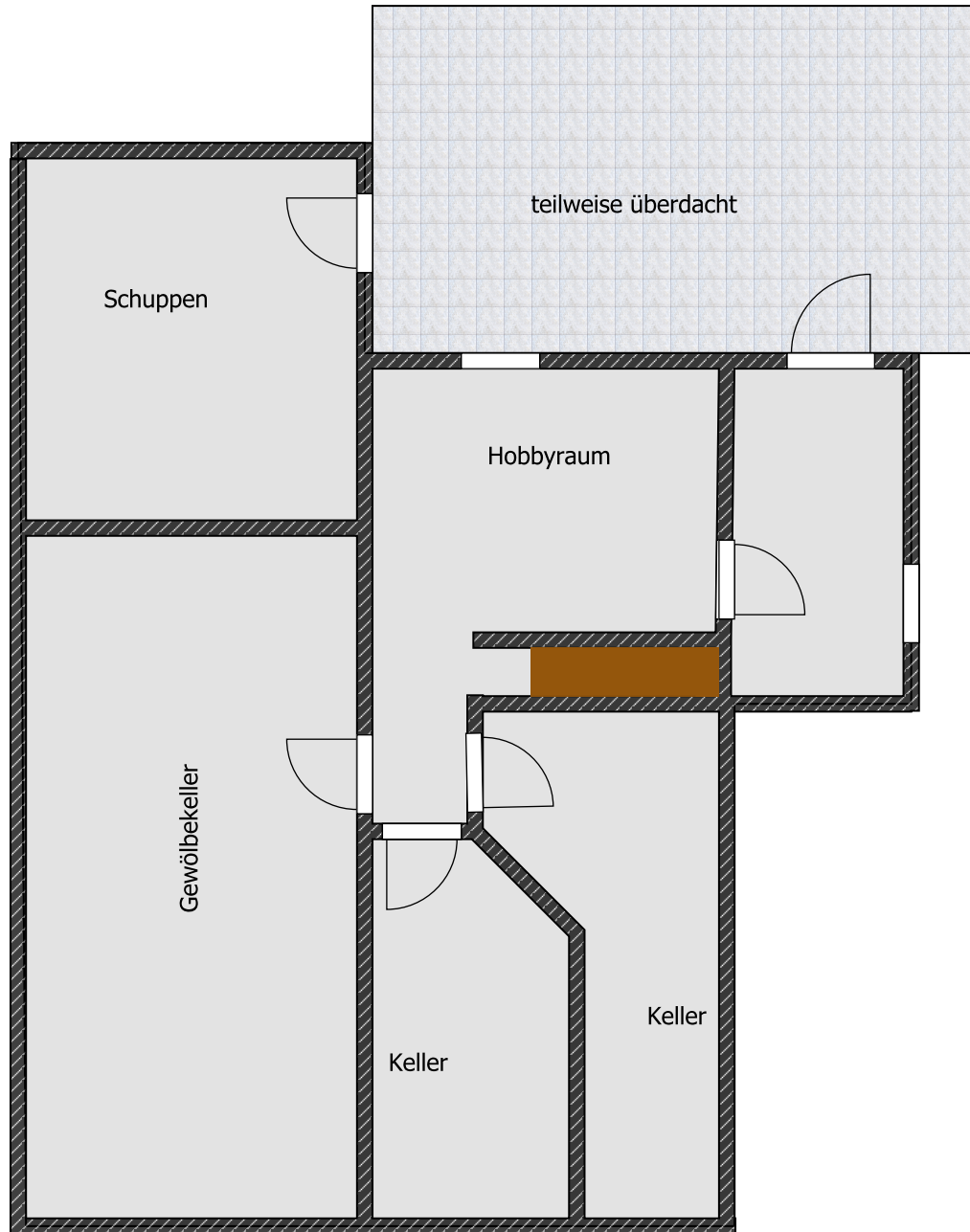
Grundriss UG (nicht maßstabsgetreu)
