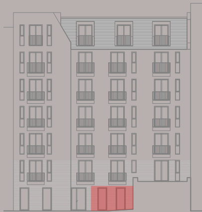
Hofansicht
