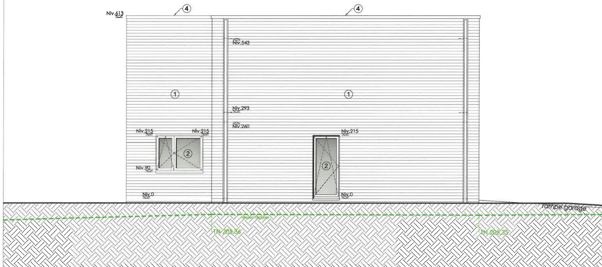
Façade Ouest - coupe dans terrain (Ech. 1%)
