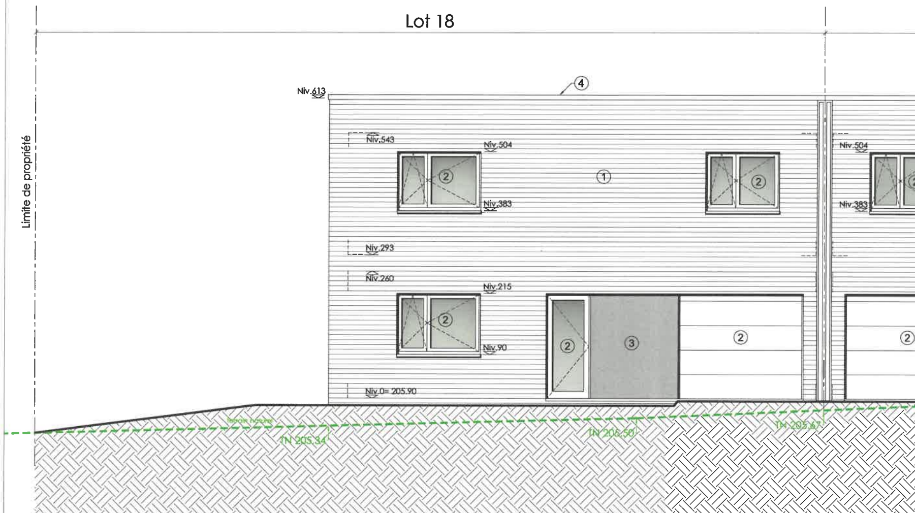
Façade Sud - lot 18 - coupe dans terrain (Ech. 1%)
