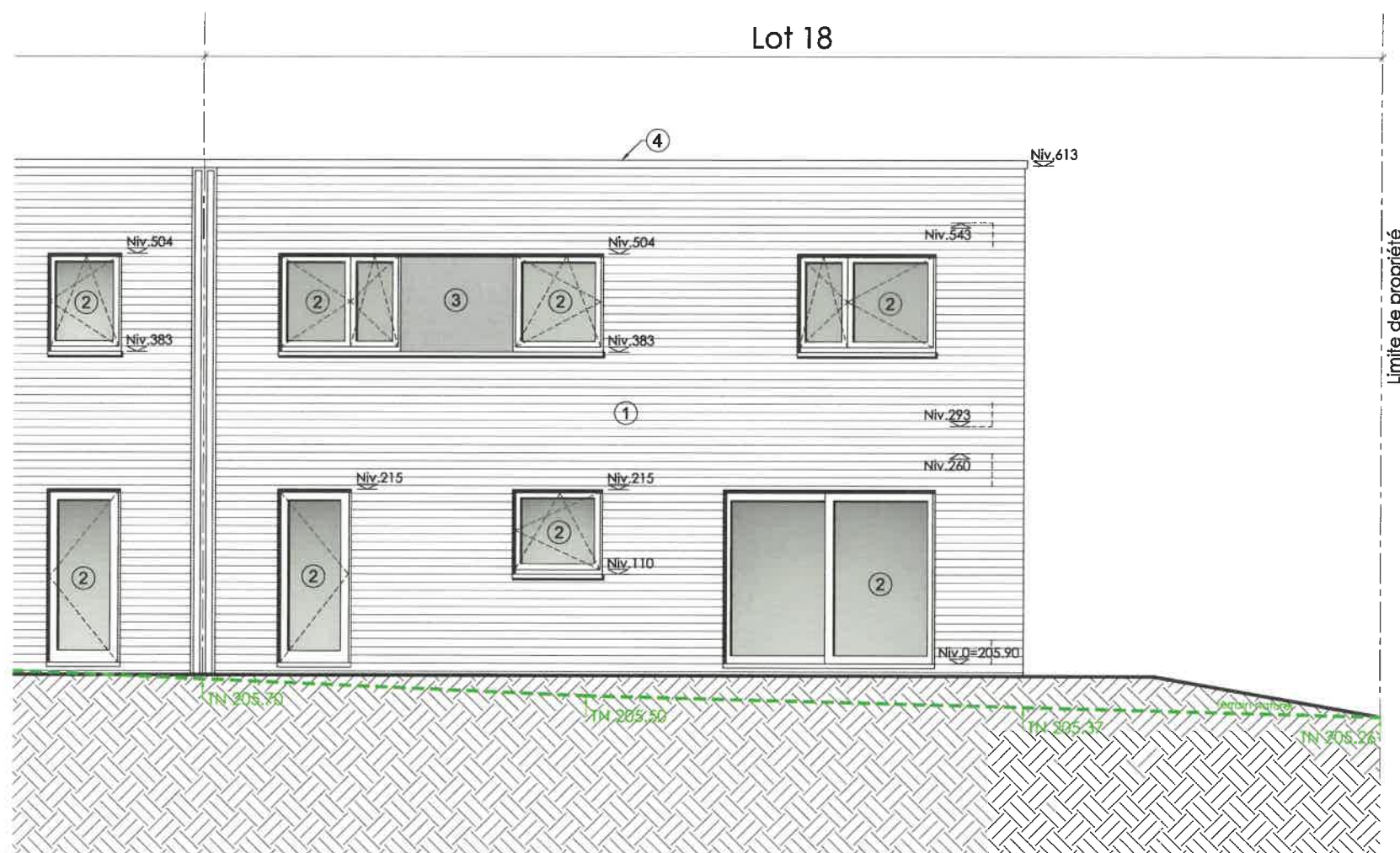
Façade Nord - coupe dans terrain (Ech. 1%)
