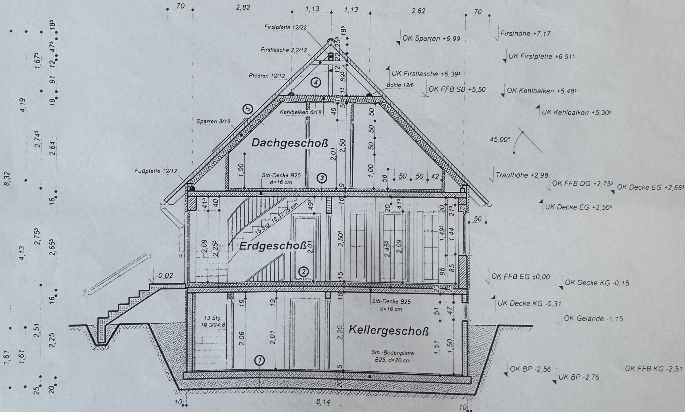
Schnitt A-A
