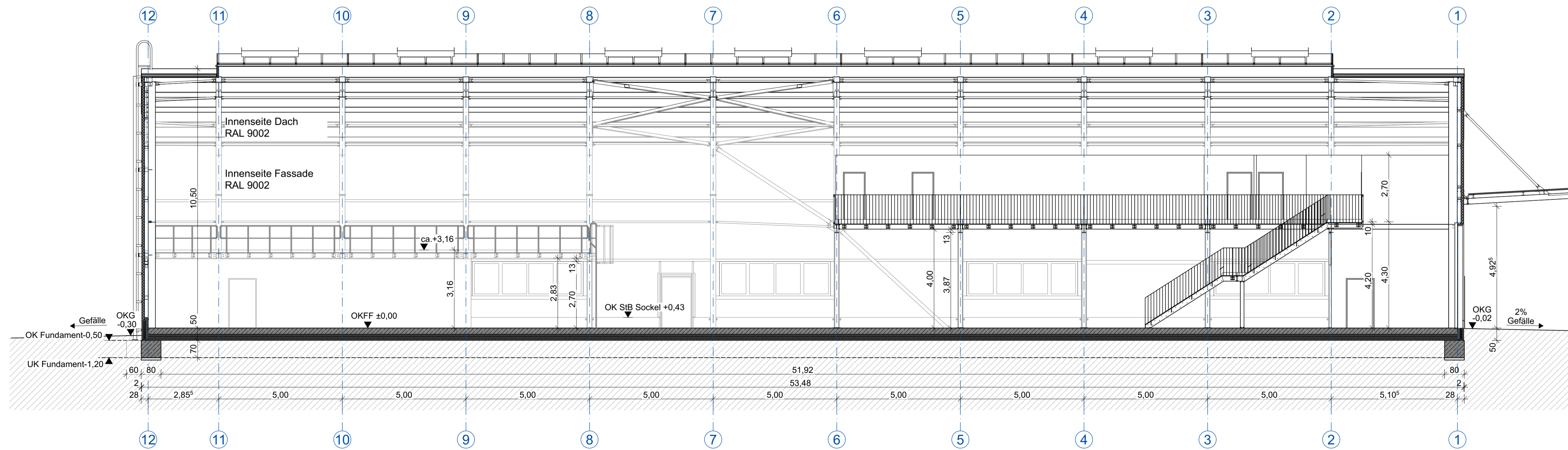
B Schnitt B-B 1:100
