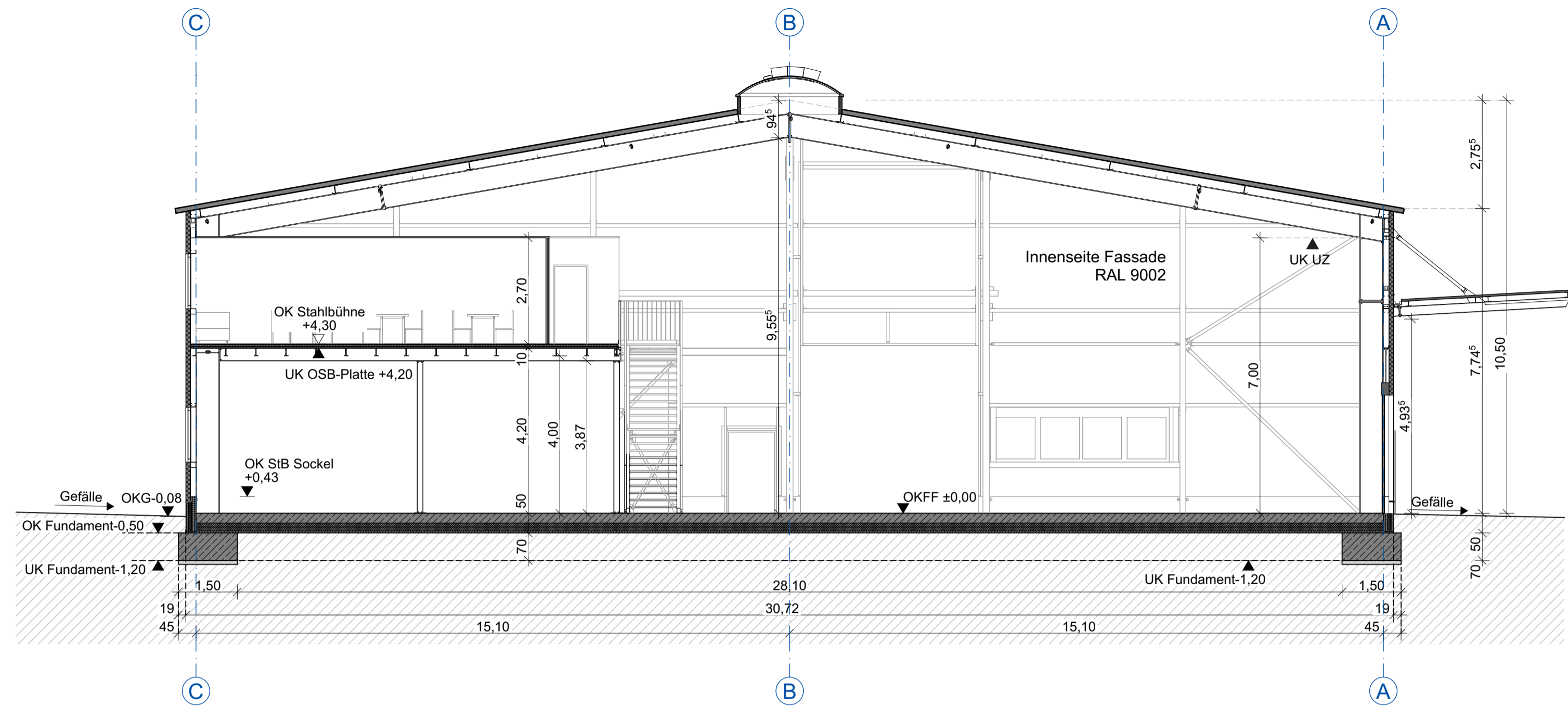
A Schnitt A-A 1:100
