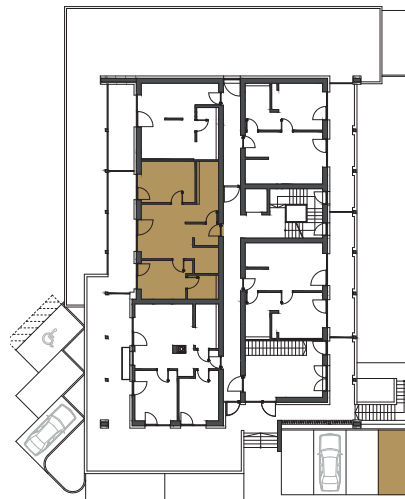
Plan Erdgeschoss
