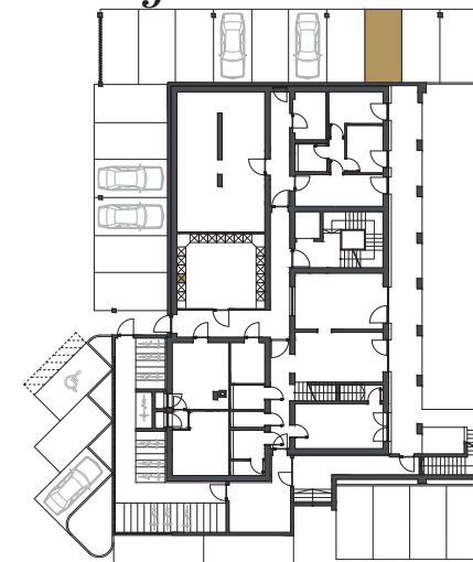
Plan Untergeschoss
